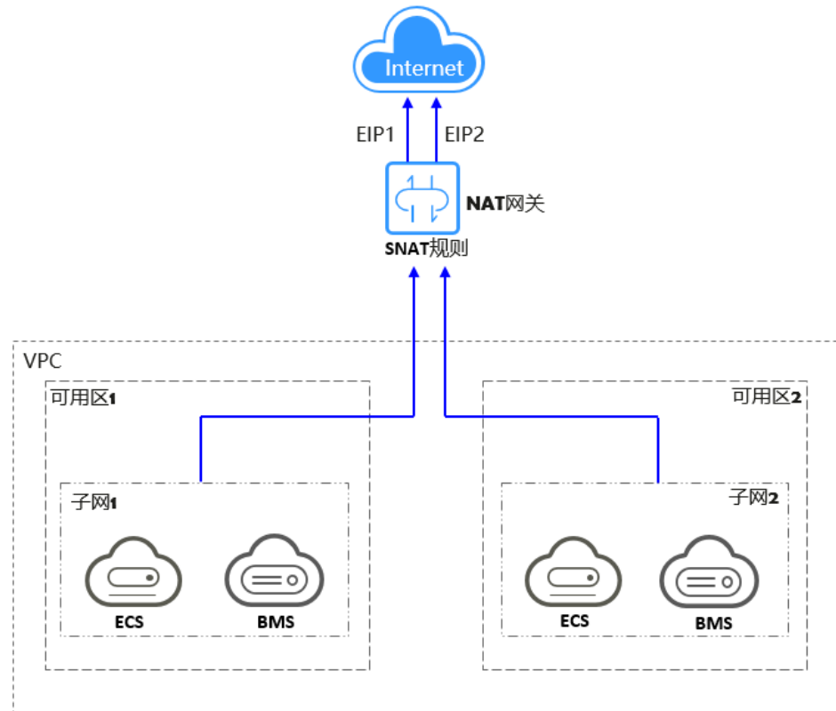
图 1-4 使用 SNAT 访问公网
