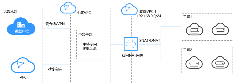
图 4-1 私网 NAT 网关
